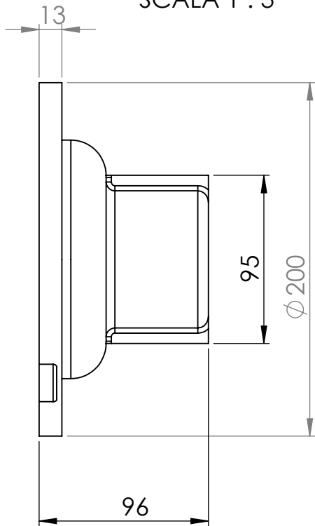
SEZIONE B-B SCALA 1 : 3
