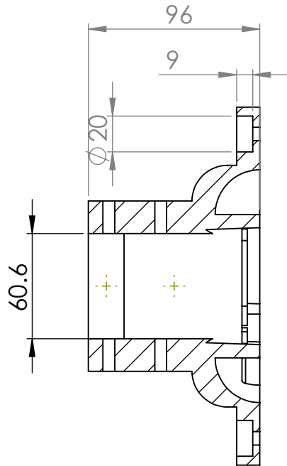
SEZIONE A-A SCALA 1 : 3
