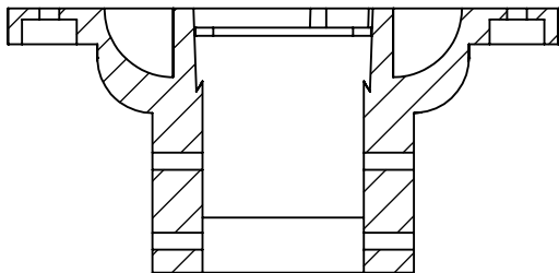
SEZIONE B-B SCALA 1 : 3
